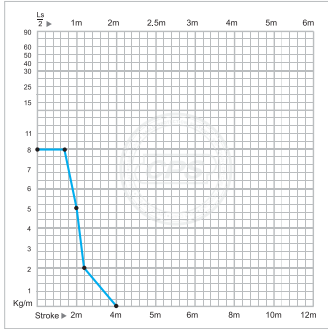
Unsupported Length Desteksiz Uzunluk Grafiği
