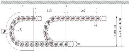
Unsupported Length Desteksiz Uzunluk Grafiği
